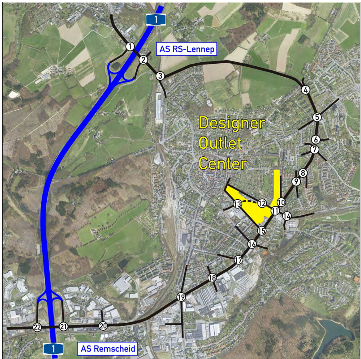
Abbildung 1: Lage des Vorhabens und untersuchte Knotenpunkte in Remscheid-Lennep (Kartengrundlage: Google Earth Pro)
